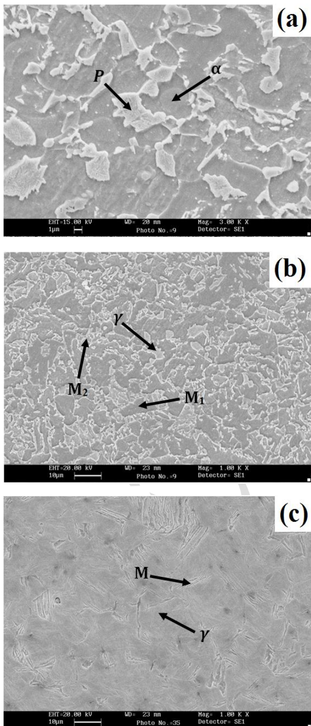
Fig. 3 SEM image of samples (a) raw, (b) Q-P-T, (c) Q-T. شکل 3 تصویر SEM از نمونه‌های (الف) خام، (ب) Q-P-T، (ج) Q-T
