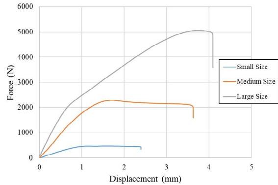
Fig. 8 Comparison of tensile force in specimens with different size. شکل 8 مقایسه نیروی تحمل شده توسط سه نمونه با سایز مختلف
