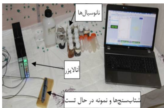
شکل 12 تجهیزات مودال و نمونه‌های نانو سیال‌های آماده سازی شده Fig. 12 The modal equipment and Nano-Fluids
