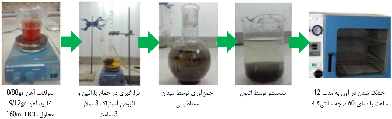
شکل 2 روند سنتز اکسید آهن
