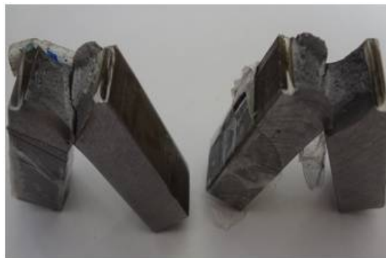
شکل 20 سطح مقطع شکست نمونه‌های آزمون ضربه
