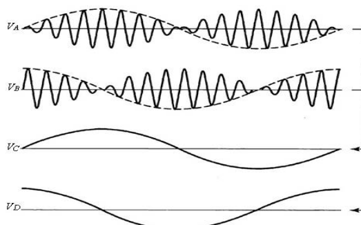
Fig. 5 Encoder output signals before and after the demodulation شکل 5 سیگنال‌های خروجی انکودر، قبل و بعد از دمدولاسیون [19]
