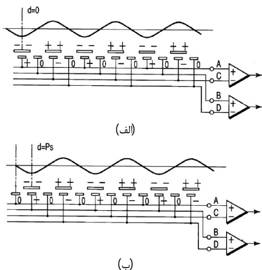
Fig. 2 Charges induction on the four-phase electrodes شکل 2 نحوه‌ی القای بار در الکترودهای چهار فاز [19]
