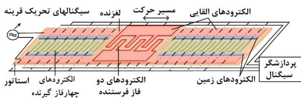
Fig. 1 Schematic diagram of the proposed capacitive encoder شکل 1 شماتیک انکودر خازنی با لغزنده نامقید
