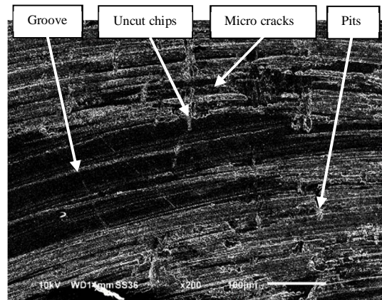
Dry machining, \times 200 (الف)
