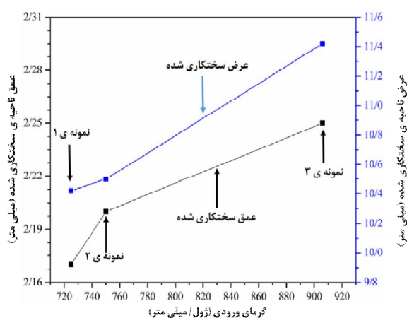
Fig. 3 Hardened area geometry for all three samples 1, 2 and 3 شکل 3 هندسه‌ی منطقه‌ی سختکاری شده برای هر سه نمونه‌ی 1، 2 و 3
